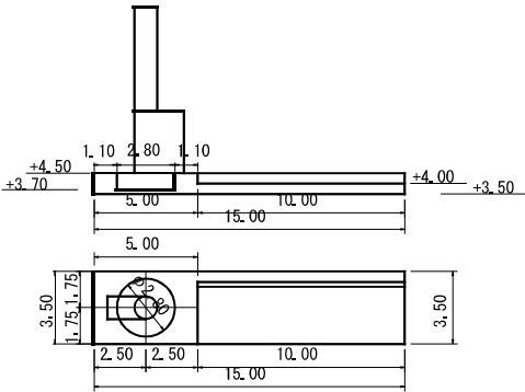
灯台基礎
