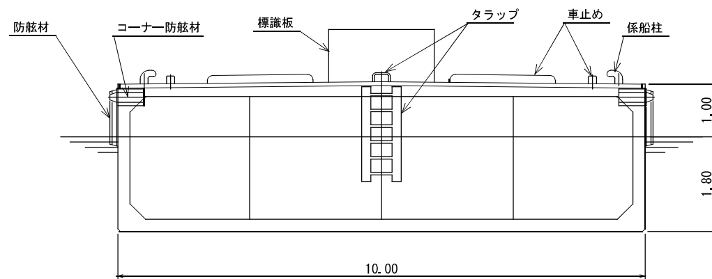
正 面 図 S = 1 / 1 0 0
