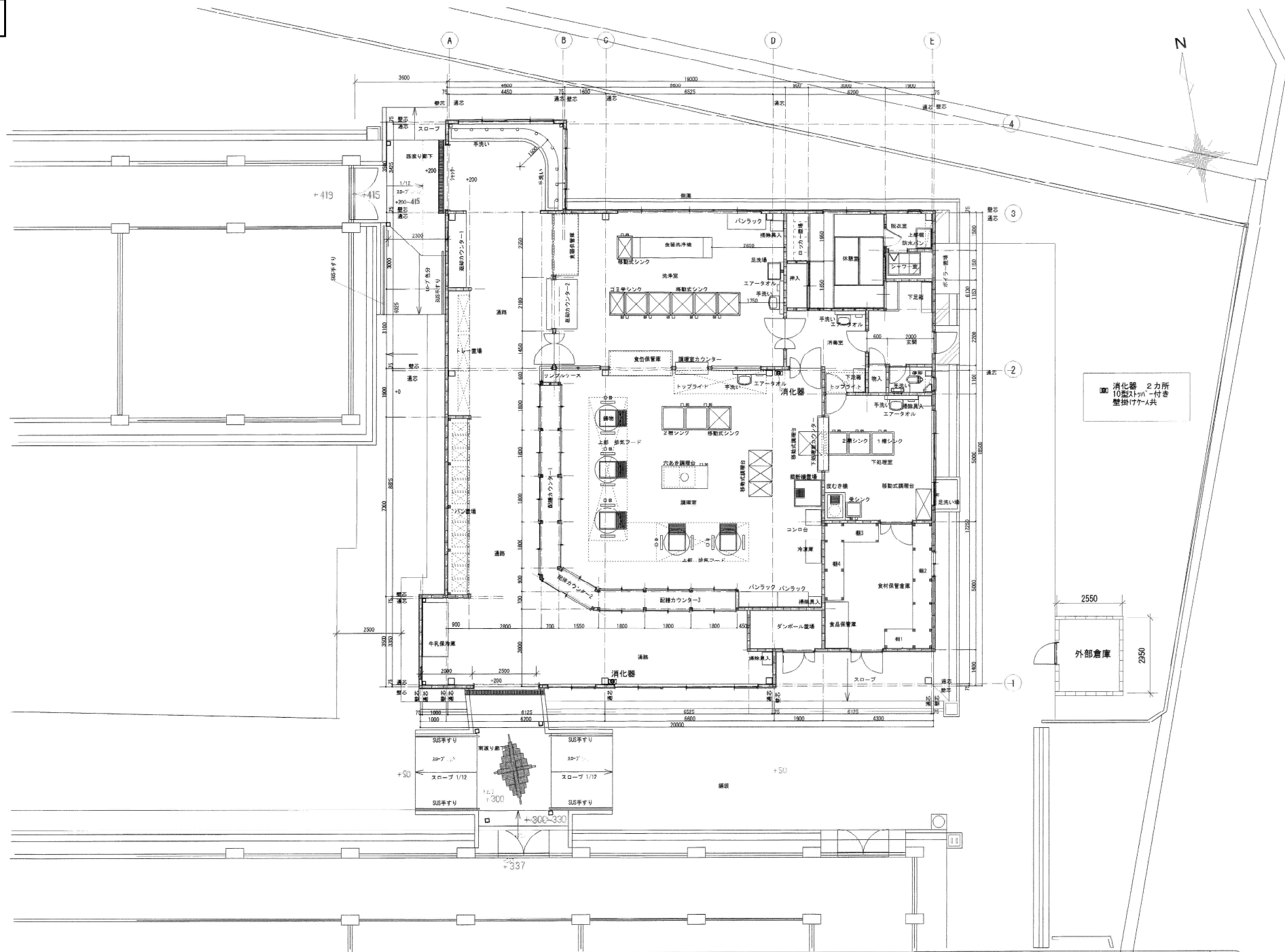
平面図 S=1/100
