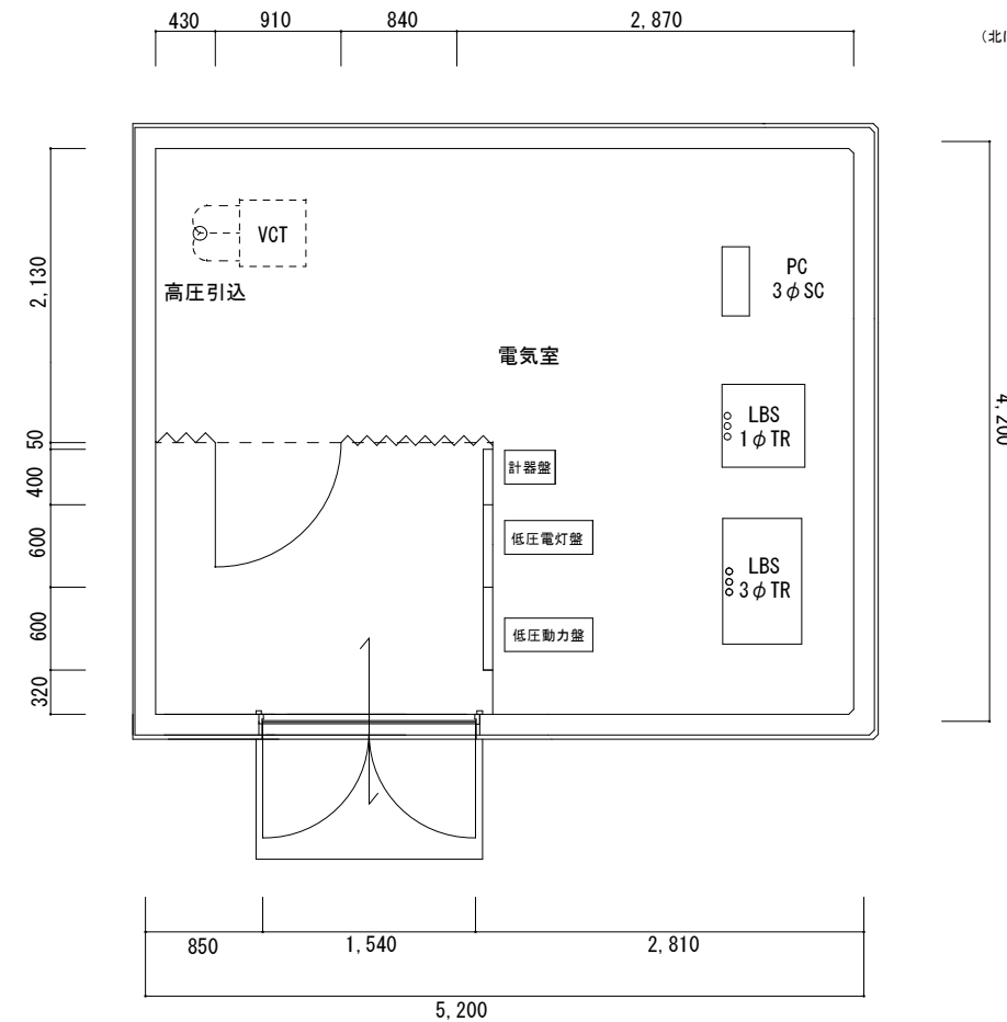
電気室平面詳細図 S=1:60
