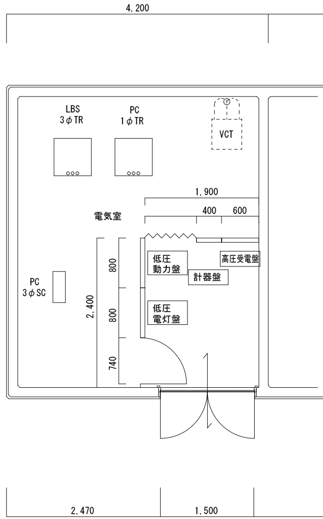
電気室平面詳細図 S=1:60
