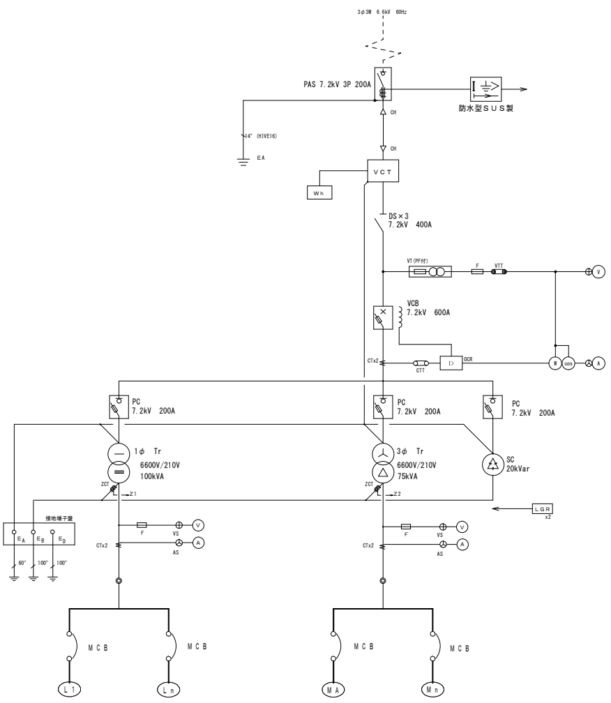
高圧受電設備単線結線図
