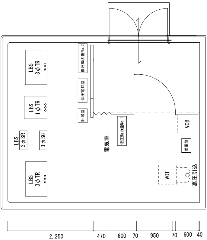
電気室平面詳細図 S=1:60
