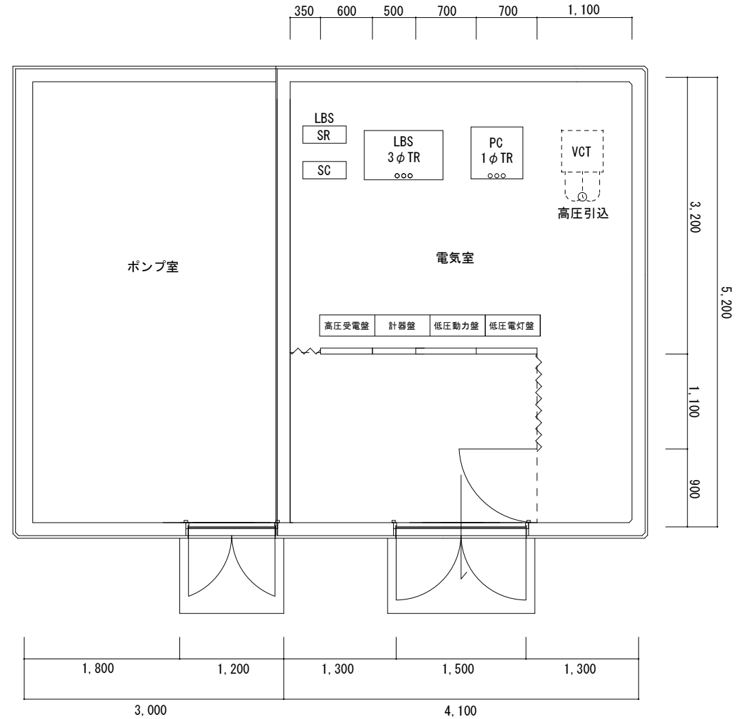
電気室平面詳細図 S=1:60
