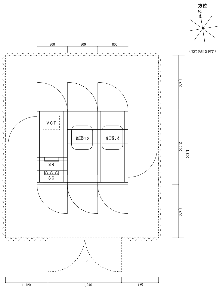
電気室平面詳細図 S=1:40
