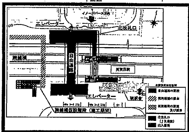
山陽本線英賀保駅自由通路整備工事 (姫路市飾磨区山崎地内外) 平面図
