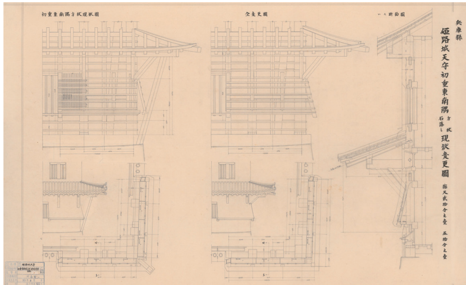
姫路城天守初重東南隅方杖石落し現状変更図
