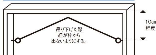
写真作品ヒートンおよび紐取り付け図(例)
